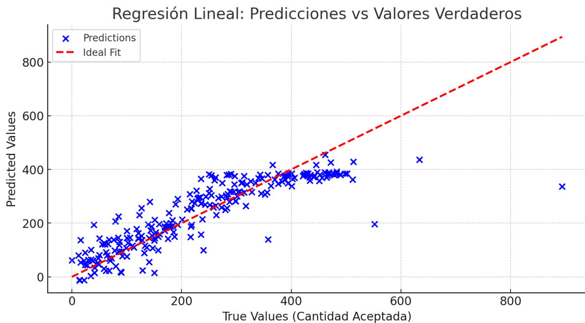
Figura 3: muestra las predicciones del modelo frente a los valores reales. La línea roja representa una predicción perfecta, y los puntos azules muestran las predicciones realizadas por el modelo.
