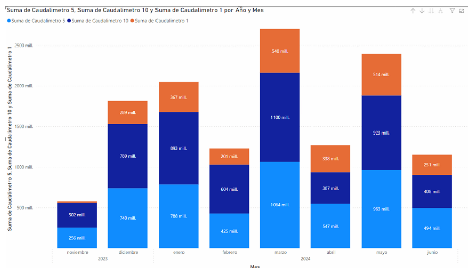
Figura 3. Caudalímetros que totalizan el agua extraída de pozo
