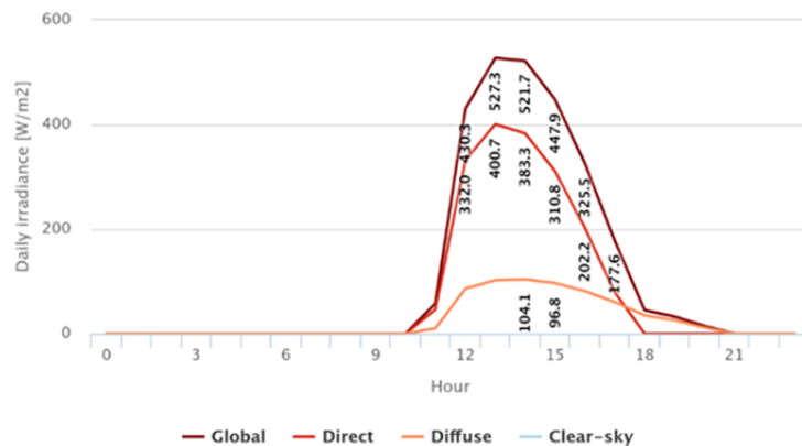
Figura 4: Irradiancia media por hora en W/m^2 - Caso 1: Azimut 120
