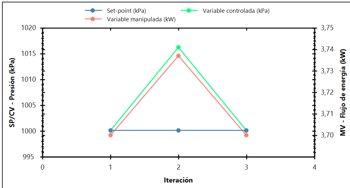
Figura 2. Iteraciones vs Set- point, Variable manipulada, Variable controlada. Copia de la pantalla simulador
