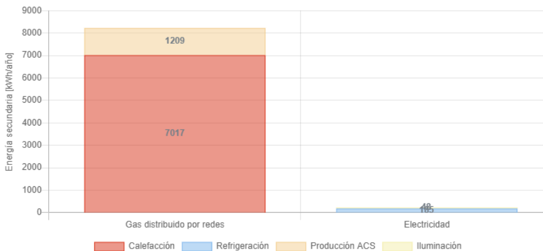
Figura 24. Detalle de requerimiento de energía secundaria Modelo Mampostería.
