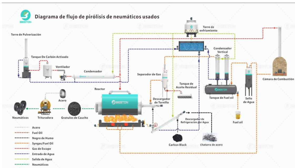
Figura 6: Diagrama de proceso
