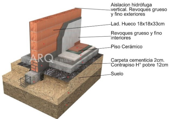
Fig.10. Detalle envoltante modelo Mampostería Fig.11. Detalle envoltante modelo Mampostería c/aislación Fuente: Edición propia de imágenes tomadas de https://arqaldetalle.com .
