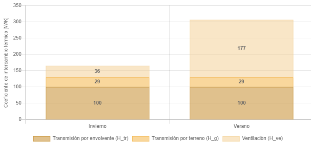
Figura 15. Coeficientes globales de intercambio térmico Modelo Mamposería c/aislación.
