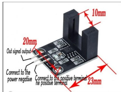
Fig. N°6: Sensor de rpm LM393
