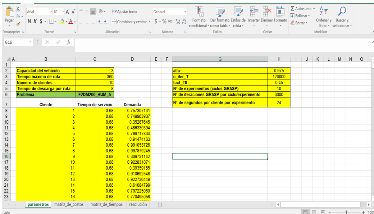
Figura 2 Ingreso de parámetros relacionados con el recocido simulado y el problema.
