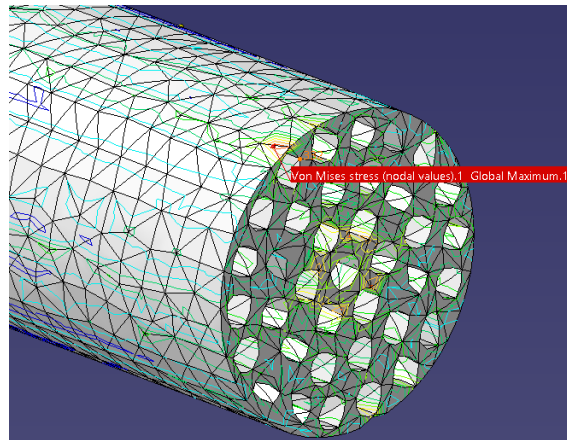
Figura 4. Modelado por elementos finitos de las tensiones en la estructura de fundición GRP400 del canister en CATIA V5
