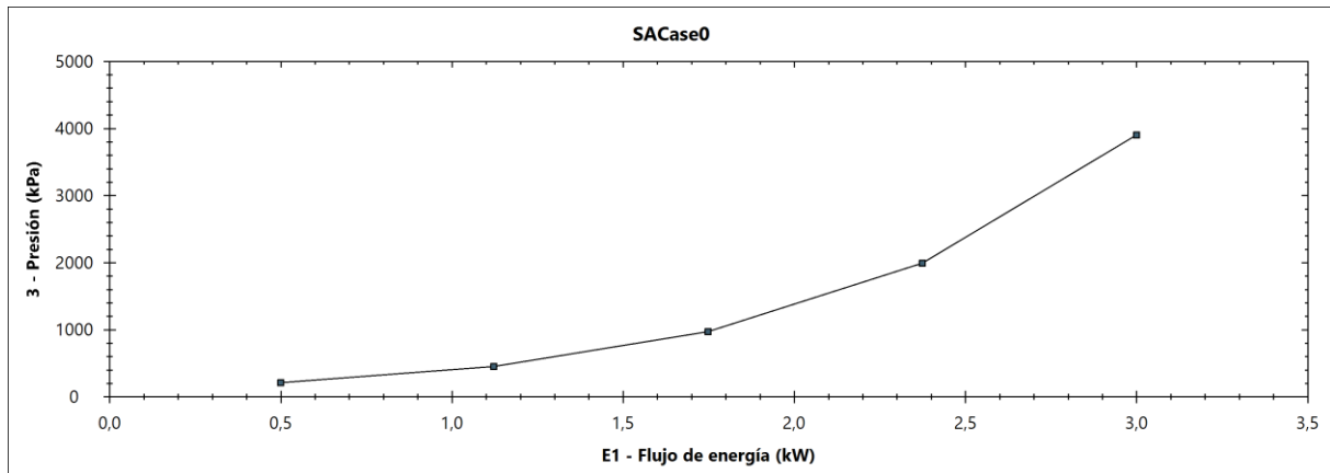
Figura 3. Flujo de energía vs Presión. Copia de la pantalla del simulador
