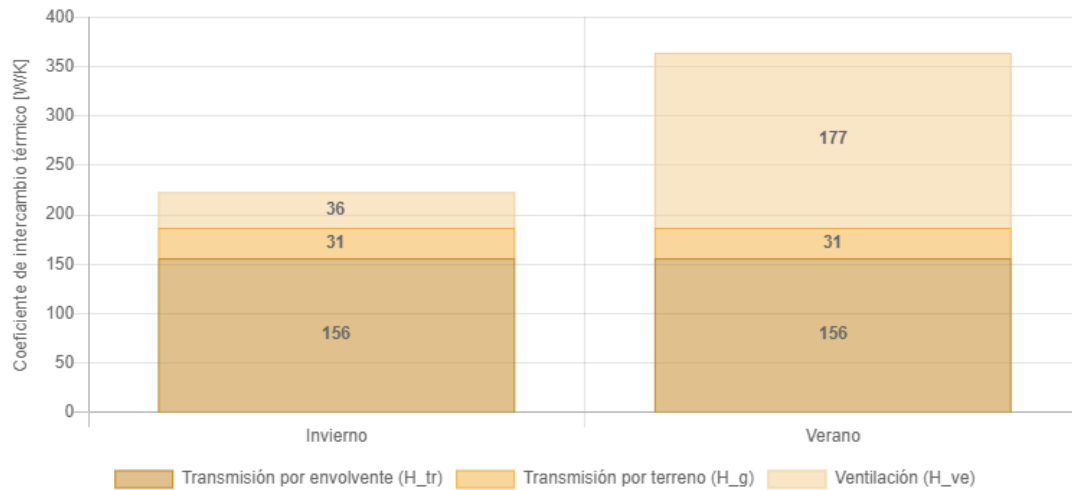
Figura 14. Coeficientes globales de intercambio térmico Modelo Mamposería.
