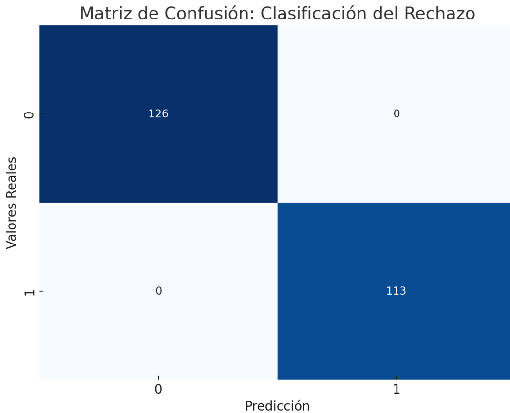
Figura 4: matriz de confusión sobre el rendimiento del modelo de clasificación, con una separación perfecta entre predicciones correctas y reales en ambos casos (rechazo bajo y rechazo alto).
