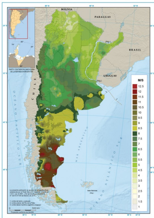
Figura 3. Potencial energético eólico
