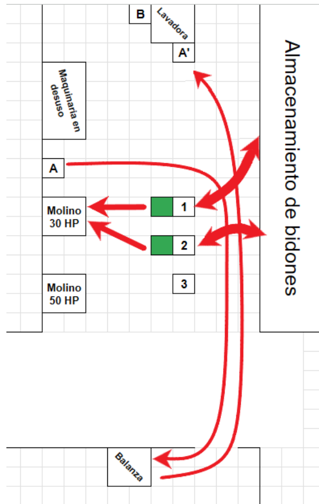
Figura 5 - Layout del proceso de molido y circulación de material.
