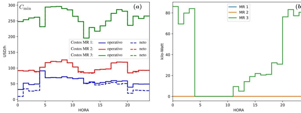
Figura 14 Operación en invierno con generación fotovoltaica. (a) Costos operativos y netos; (b) Importaciones.
