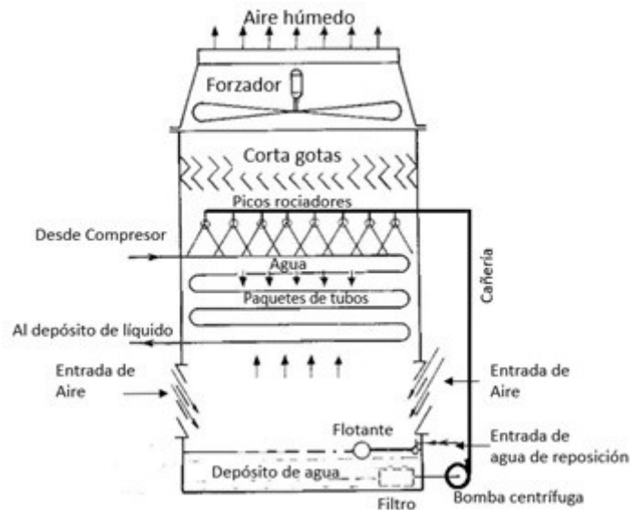
Figura N° 1. Bomba en Condensador evaporativo de serpentines
