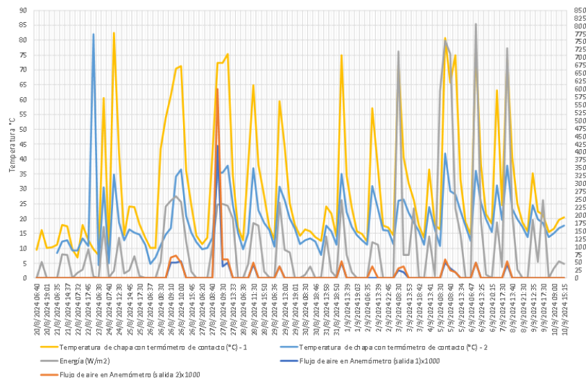
Figura 14: Temperatura de la chapa del panel, flujo de aire y energía solar, medición de invierno
