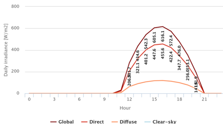
Figura 6: Irradiancia media por hora en W/m^2 - Caso 2: Azimut 180
