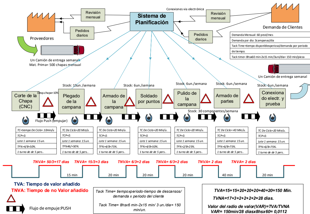
Figura 5. Diagrama de Flujo de Valor (VSM) para la fabricación de campanas extractoras.
