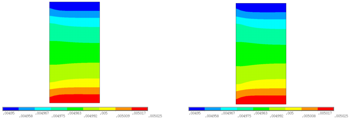
Figura 5 Contornos de deformación total en el plano de simetría yz para el material 1 (izq.) y 2 (der.) para la geometría 1 para el estado final de carga investigado
