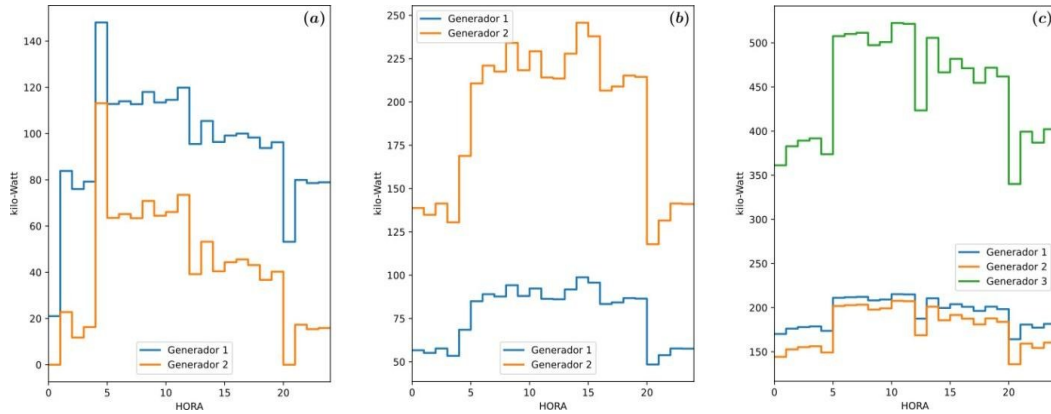
Figura 10 Generación para invierno en modo interconectado. (a) Industria 1; (b) Industria 2; (c) Industria 3.
