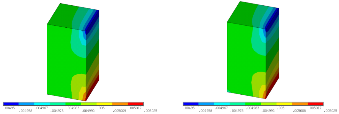
Figura 3 Contornos de deformación total para el material 1 (izq.) y 2 (der.) para la geometría 1 para el estado final de carga investigado
