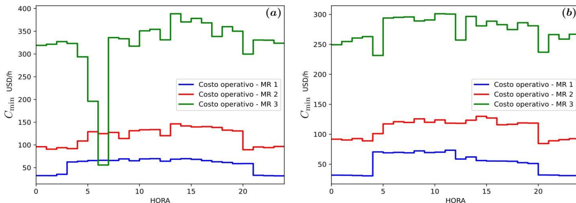
Figura 4 Costo operativo global optimizado por MR y estación en modo isla. (a) verano; (b) invierno.
