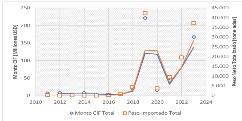
Figura 9 - Totalizado Módulos Solares
