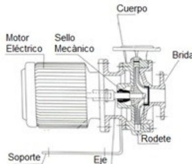
Figura N° 2. Partes principales de la bomba centrífuga.
