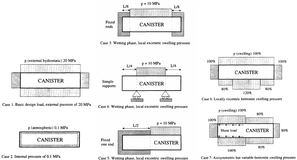
Figura 2. Condiciones de carga (POSIVA)
