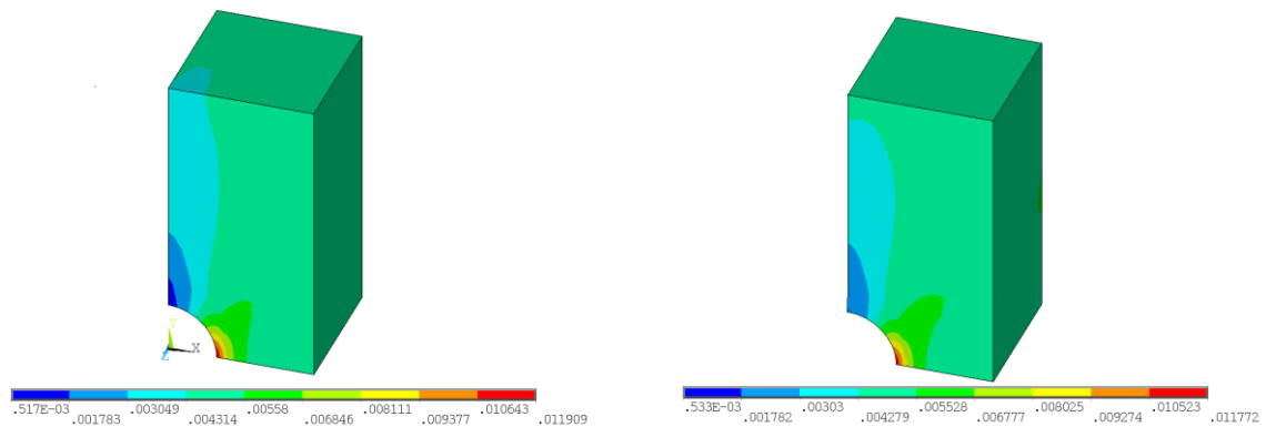
Figura 4 Contornos de deformación total para el material 1 (izq.) y 2 (der.) para la geometría 2 para el estado final de carga investigado
