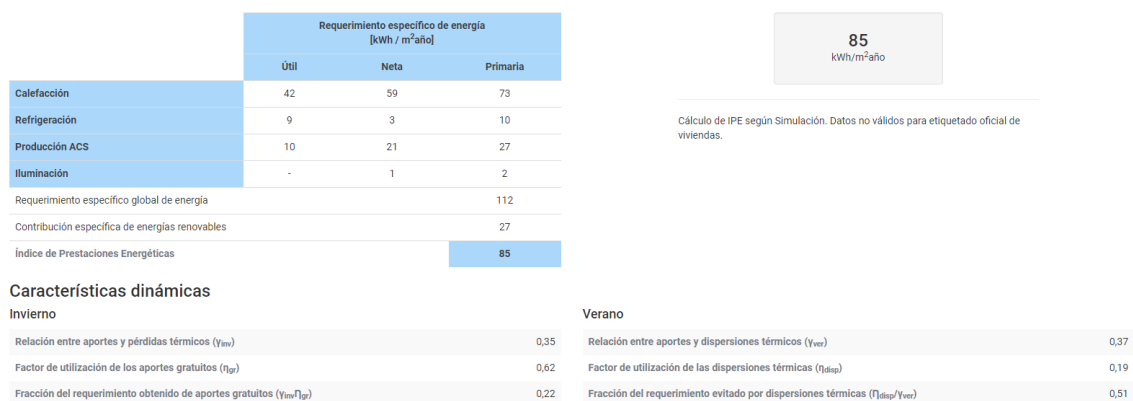
Figura 20. Prestaciones energéticas Modelo Madera.
