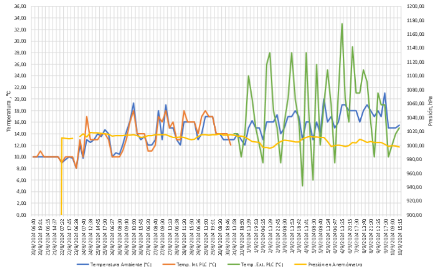
Figura 13: Temperatura interna (local), externa y presión atmosférica
