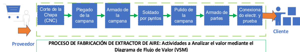
Figura 4. Diagrama de bloque del proceso de Fabricación de Campanas de extracción de aire. Fuente: Elaboración propia.
