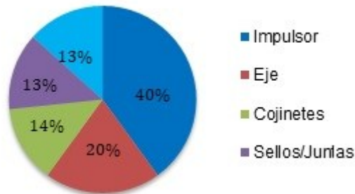
Figura N° 4. Modos de fallas por componente.
