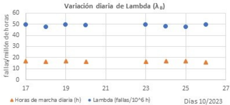
Figura N° 7. Datos de tasa instantánea de fallas ( \lambda ).
