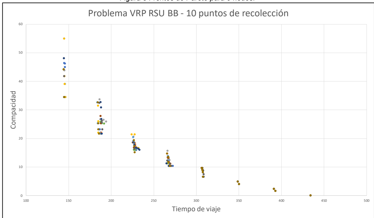
Figura 4 Frentes de Pareto para 10 nodos.
