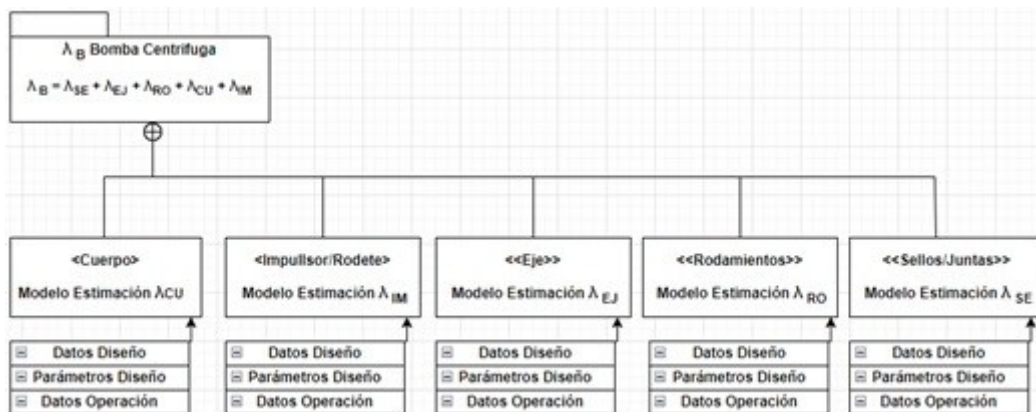
Figura N° 10. Diagrama UML de módulos de software.
