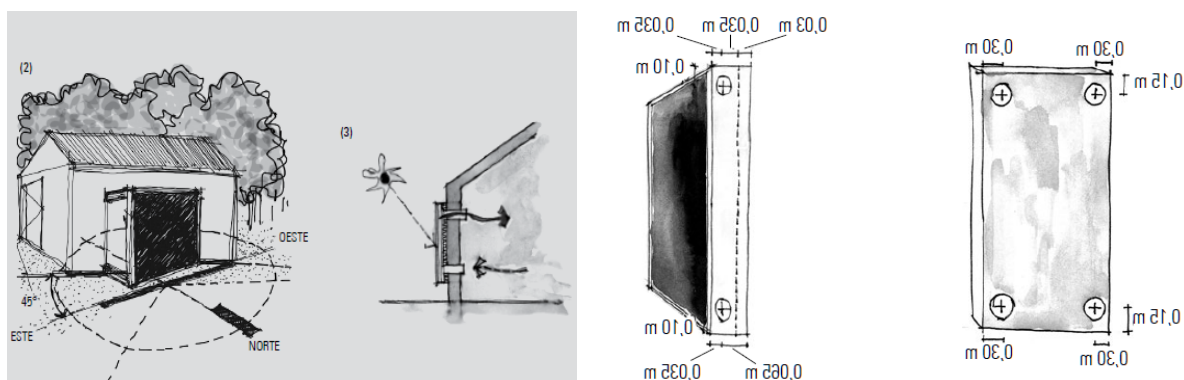
Figura 8: Calefactor solar IIPAC FAU UNLP – CONICET, disposición y dimensiones
