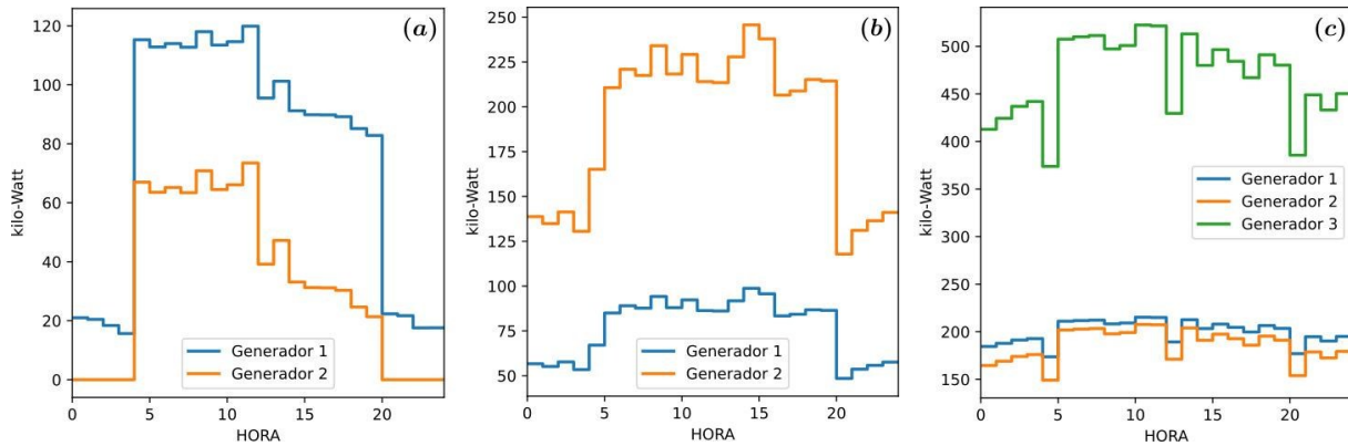
Figura 6 Despacho de generadores para invierno en modo isla. (a) Industria 1; (b) Industria 2; (c) Industria 3.
