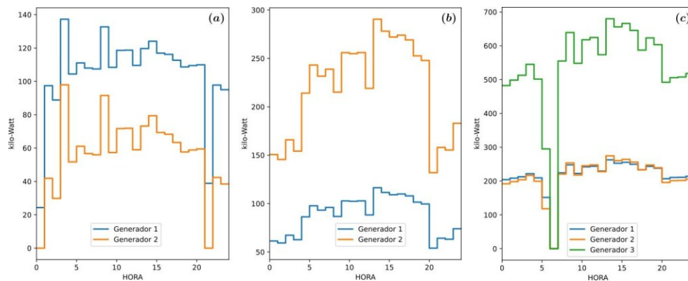
Figura 8 Generación para verano en modo interconectado. (a) Industria 1; (b) Industria 2; (c) Industria 3.
