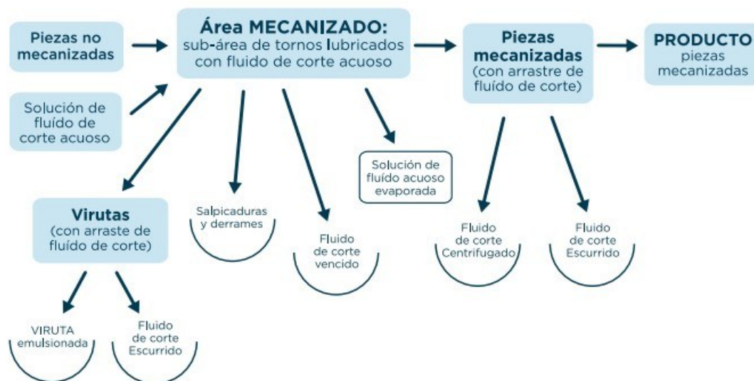
Figura 1. Diagrama de flujo de fluidos de corte. Fuente: Secretaría de ambiente y desarrollo sustentable (2019).
