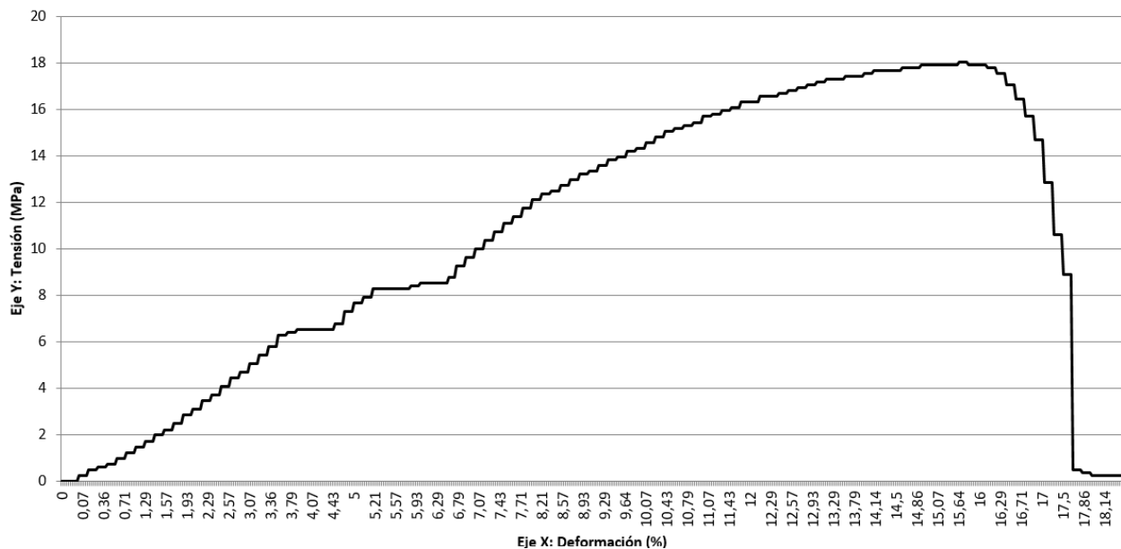
Figura 14 Ensayo de tracción de probeta Roja
