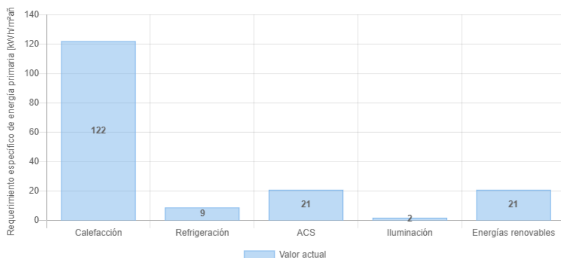
Figura 17. Requerimiento específico de energía primaria Modelo Mamposería.
