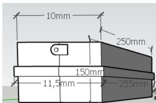
Figura 2 Representación del molde utilizado para realizar briquetas.
