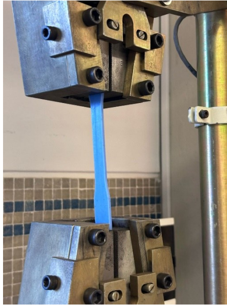
Figura 10 Ensayo de tracción
