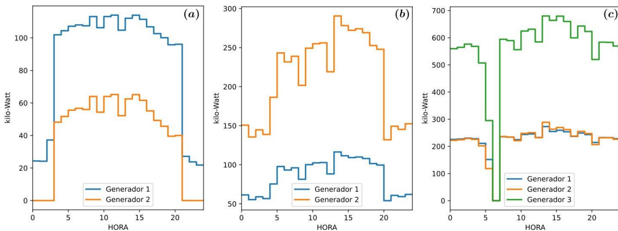
Figura 5 Despacho de generadores para verano en modo isla. (a) Industria 1; (b) Industria 2; (c) Industria 3.
