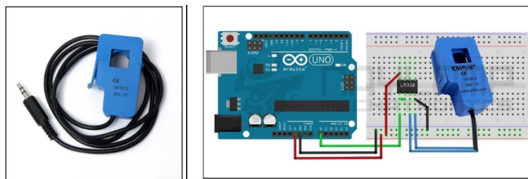
Fig. N°4: Sensor de corriente no invasivo
