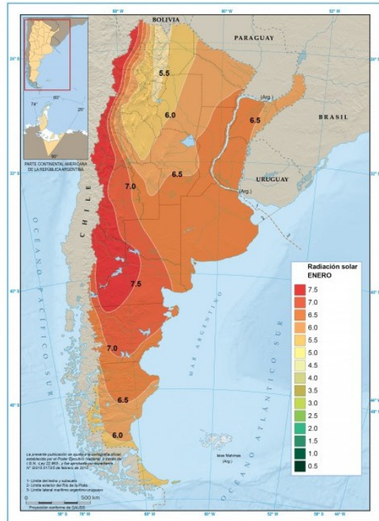
Figura 4. Potencial energético solar
