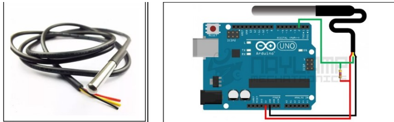
Fig. N°4: Sensor de temperatura DS18B20
