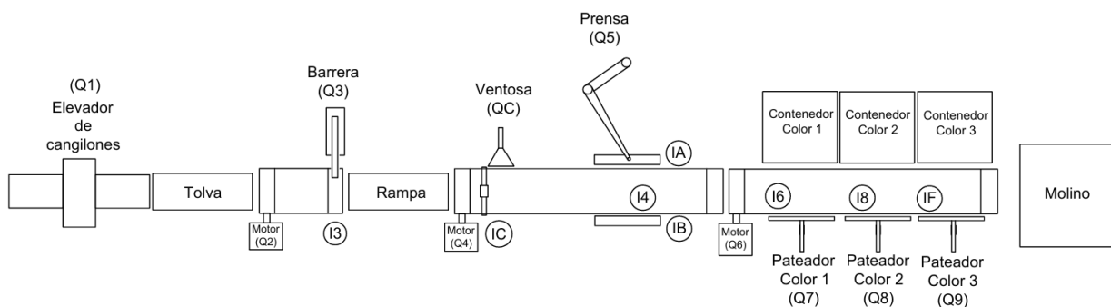
Figura 11 - Vista de planta del croquis ilustrativo
