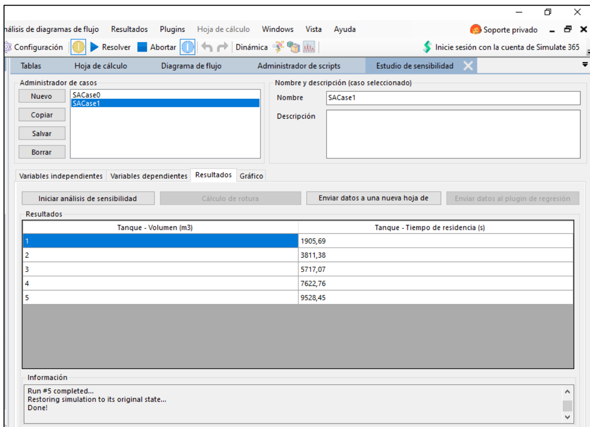
Figura 4. Tabla Volumen del tanque vs Tiempo de residencia. Copiado de pantalla simulador
