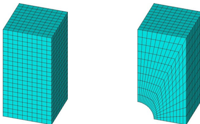
Figura 2 Mallas de elementos finitos para ambas geometrías.
