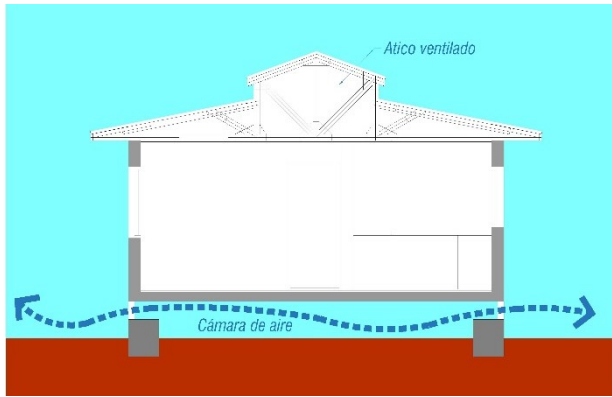
Figura 6. Corte transversal de la vivienda
