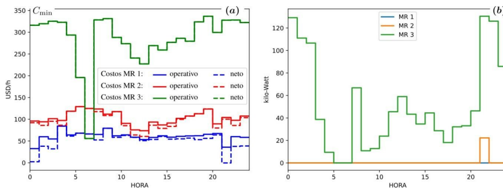
Figura 12 Operación en verano con generación fotovoltaica. (a) Costos operativos y netos; (b) Importaciones.
