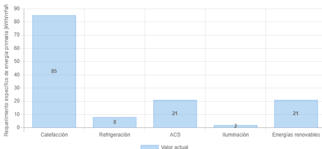
Figura 18. Requerimiento específico de energía primaria Modelo Mamposería c/aislación.
