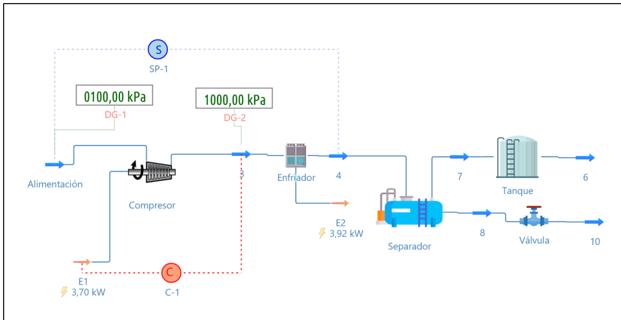
Figura1: Diagrama de flujo (Flow sheet) del proceso simulado. Copia de la pantalla del simulador
