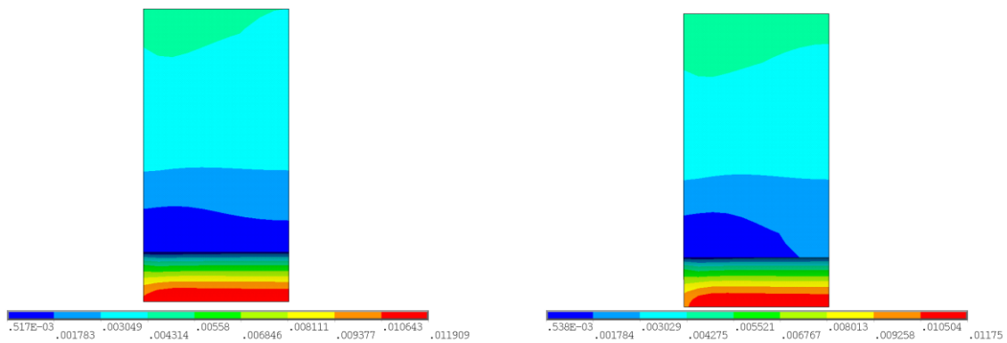
Figura 6 Contornos de deformación total en el plano de simetría yz para el material 1 (izq.) y 2 (der.) para la geometría 2 para el estado final de carga investigado
