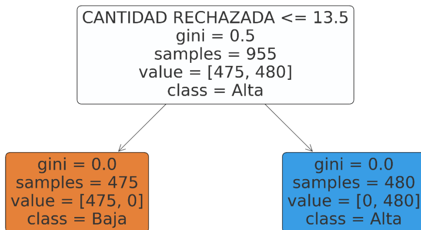
Árbol de Decisión - Clasificación de Rechazos
