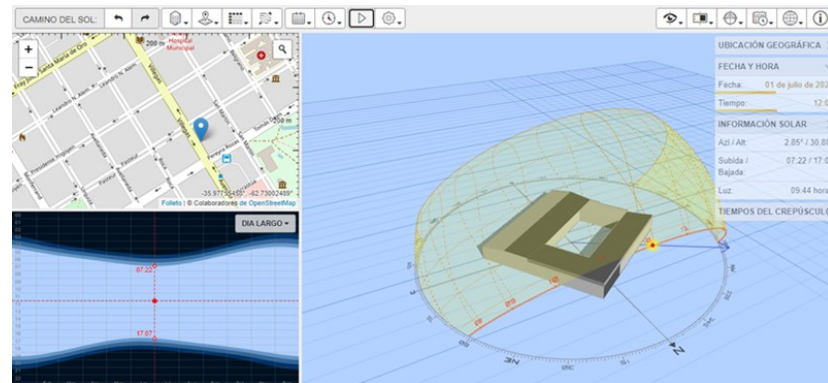
Figura 2: Incidencia solar en el muro interno
