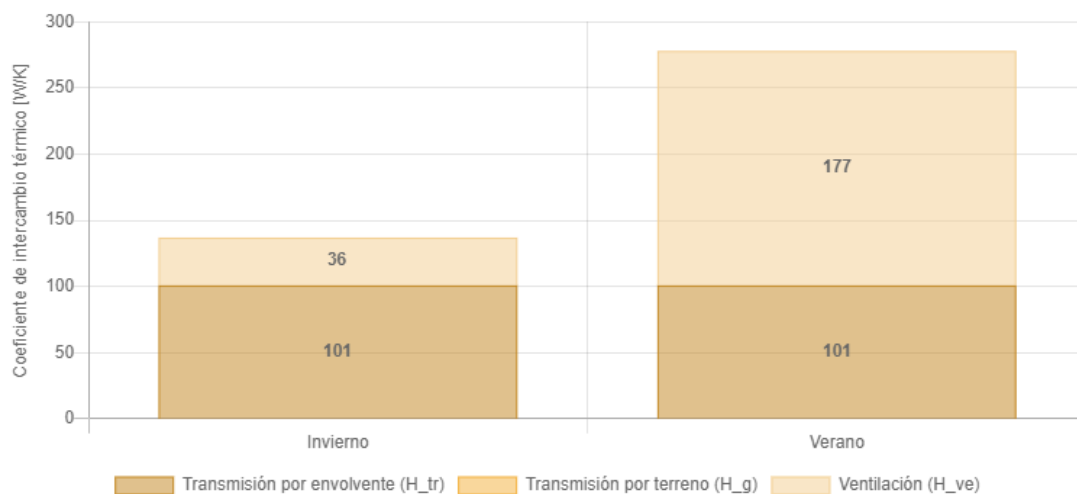
Figura 13. Coeficientes globales de intercambio térmico Modelo Madera.
