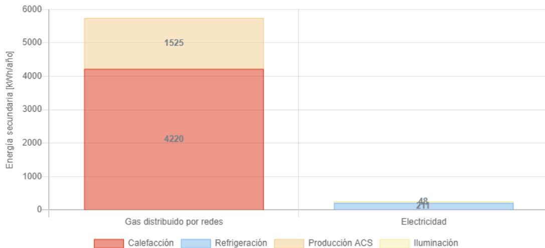
Figura 23. Detalle de requerimiento de energía secundaria Modelo Madera.
