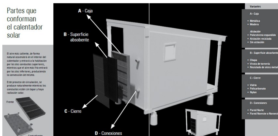
Figura 7: Sistema del calefactor solar IIPAC FAU UNLP - CONICET
