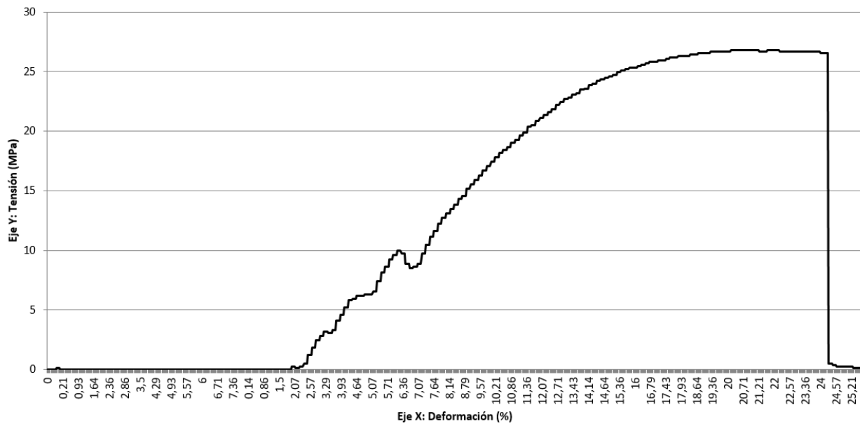
Figura 12: Ensayo de tracción de probeta Celeste
