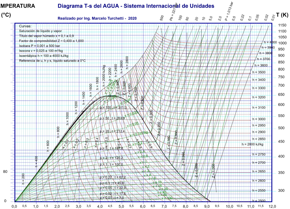
Figura 4. Diagrama Temperatura-Entropía del Agua en papel.
