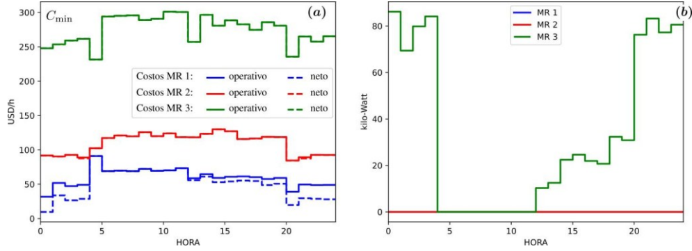
Figura 9 Operación por MR en invierno (modo interconectado). (a) Costos operativos y netos; (b) Importaciones.
