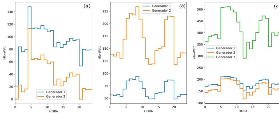
Figura 15 Despacho en invierno con generación fotovoltaica. (a) Industria 1; (b) Industria 2; (c) Industria 3.
