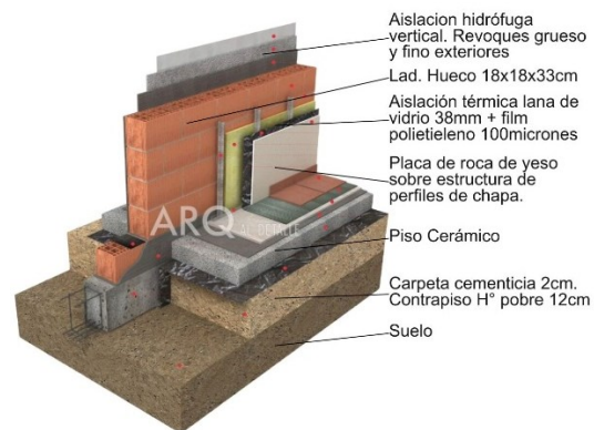
Fig.10. Detalle envoltante modelo Mampostería Fig.11. Detalle envoltante modelo Mampostería c/aislación Fuente: Edición propia de imágenes tomadas de https://arqaldetalle.com .
