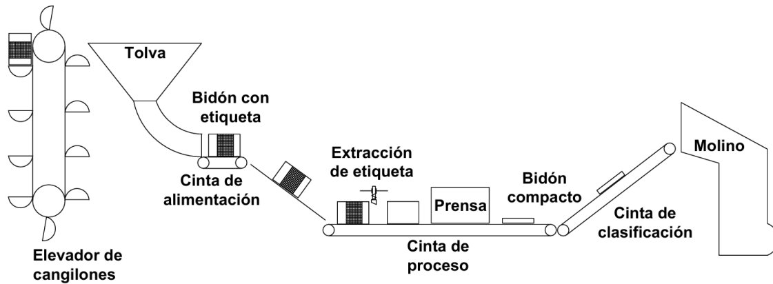
Figura 10 - Croquis ilustrativo de la procesadora de bidones.
