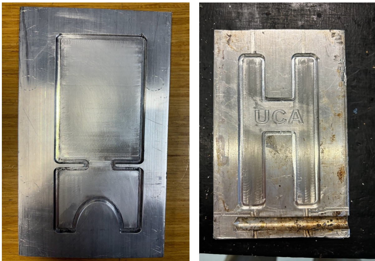
Figura 4 y 5: Matriz portacelular
