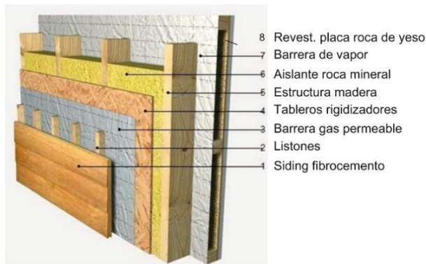
Figura 8. Detalle envolvente vertical Fuente: Edición propia de imagen de internet.
