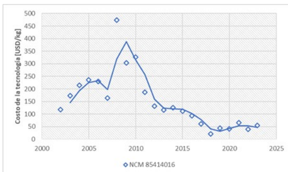
Figura 10 - Costo de la tecnología, Células Solares sin montar
