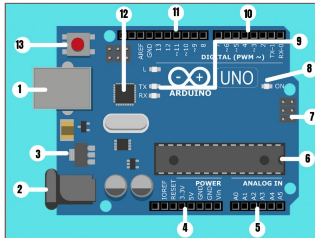
Fig. N°2: Ilustración placa Arduino UNO
