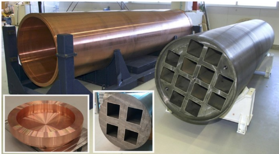
Figura 1. Componentes del canister utilizado en el sistema KBS-3
