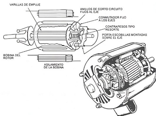
Fig. N°3: Composición de un motor AC
