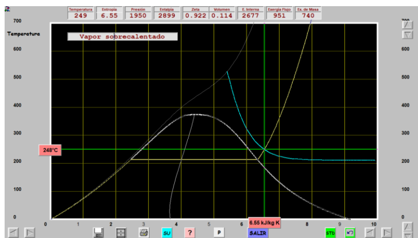
Figura 1. Vista de la pantalla del diagrama animado del vapor de agua.
