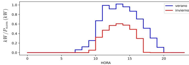
Figura 11 Producción fotovoltaica diaria para los casos simulados.
