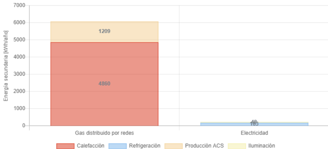
Figura 25. Detalle de requerimiento de energía secundaria Modelo Mampostería c/aislación.
