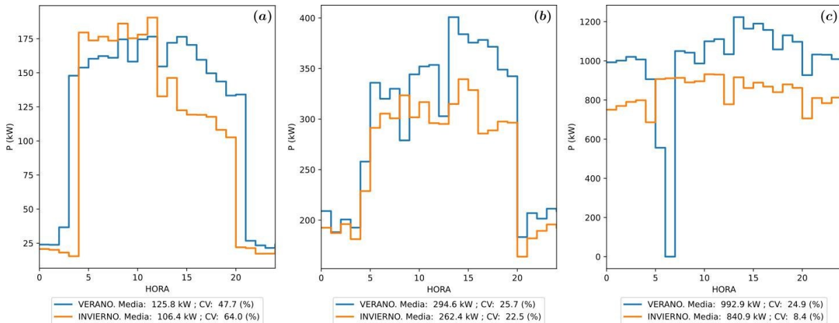
Figura 3 Demandas para un día de verano y otro de invierno. (a) Industria 1; (b) Industria 2; (c) Industria 3.
