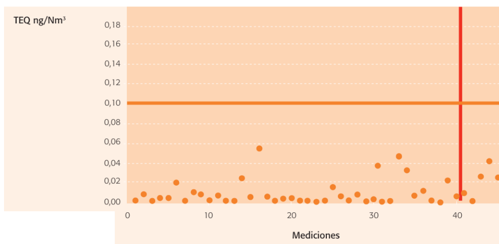
Figura 1 Emisiones de dioxinas y furanos en hornos de cemento en España en los años 2000 y 2001 versus campaña de mediciones con residuos en 2004. Fuente: Rivera & Abad (2004). Nota: TEQ significa Equivalente Tóxico Internacional.
