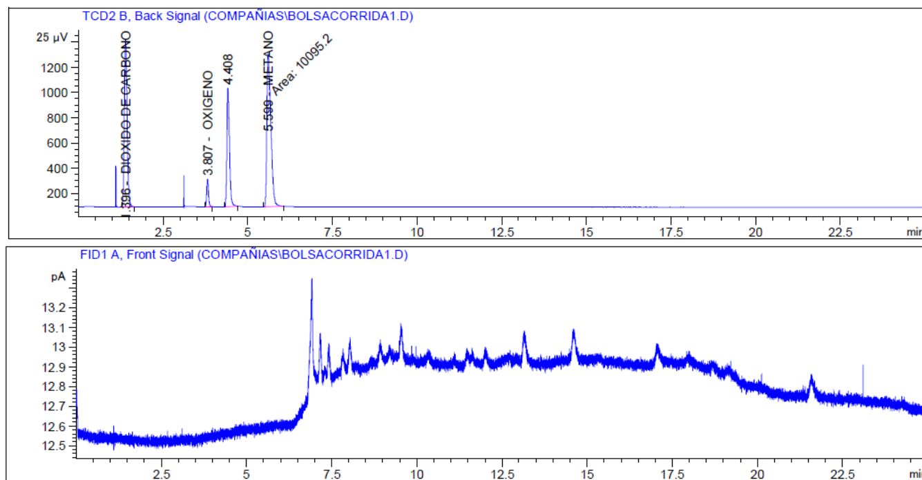
Figura 4. Cromatograma
