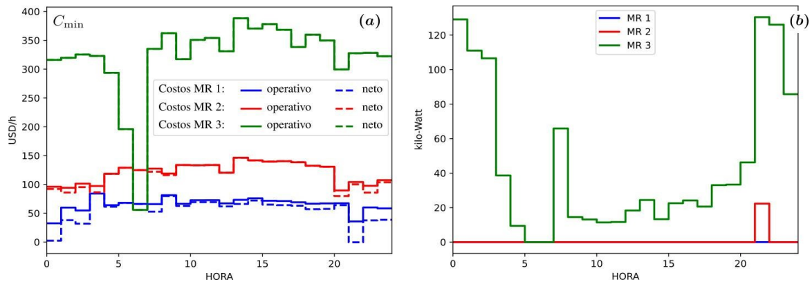
Figura 7 Operación por MR en verano (modo interconectado). (a) Costos operativos y netos; (b) Importaciones.
