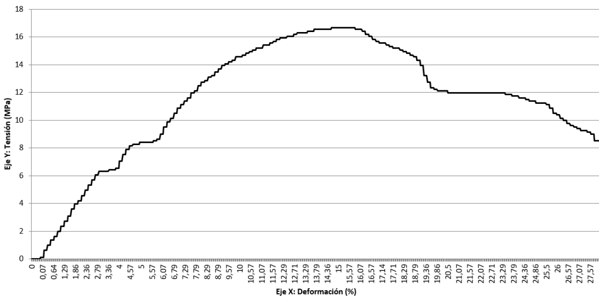
Figura 13 Ensayo de tracción de probeta Verde 2
