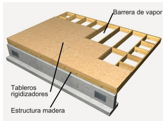
Figura 9. Detalle entrepiso Fuente: Edición propia de imagen de internet.
