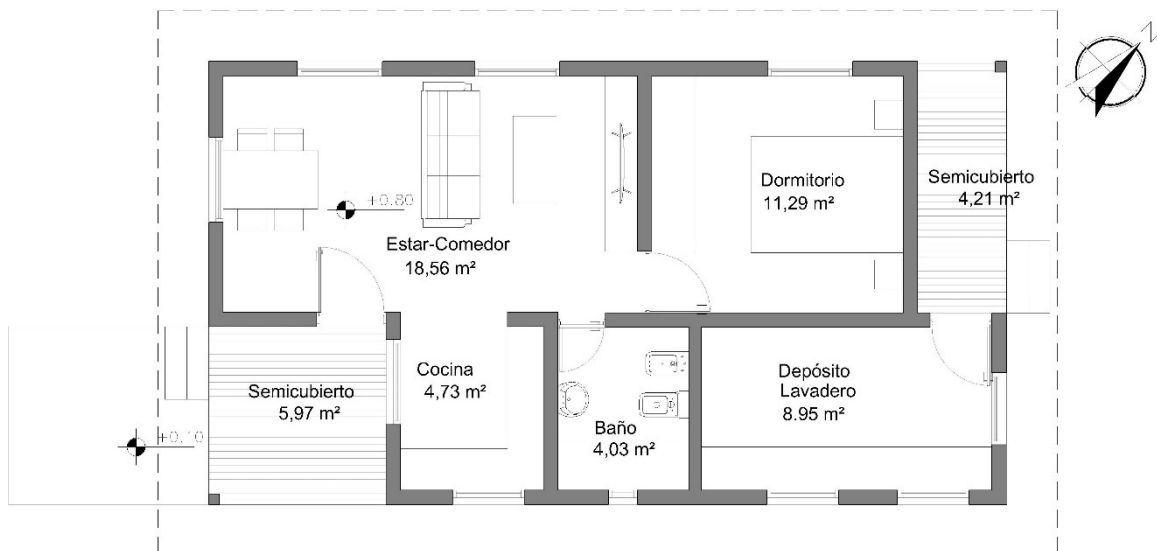
Figura 5. Planta de la vivienda del modelo evaluado.
